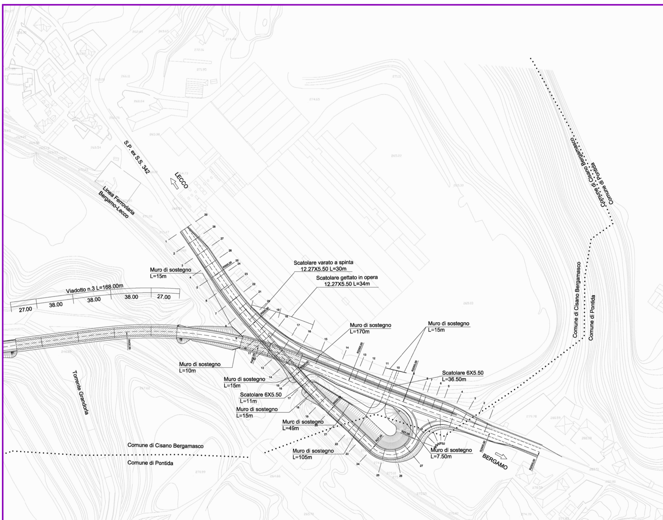
ESTRATTO PROGETTO PRELIMINARE COLLEGAMENTO DELLA VARIANTE DI CISANO BERGAMASCO E LA S.P. ex S.S.342, REDATTO DALLA PROVINCIA DI BERGAMO- SETTORE VIABILITA'- APPROVATO DALLA G.P. N. 347 DEL 30.06.2005 - 1:2.000
